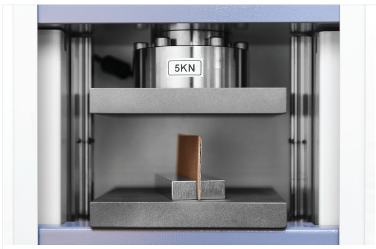
Figure: Edge Crush Test (ECT)
